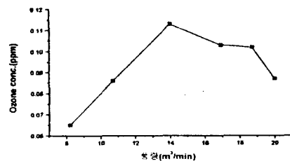
그림 2. 풍량에 따른 오존발생농도.
